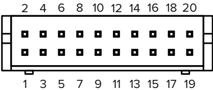
Рис. 9. Расположение контактов шлейфового разъема
