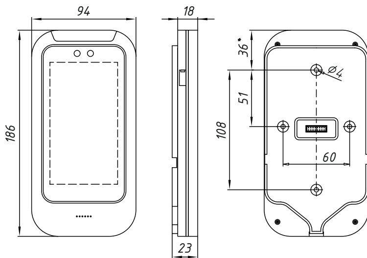
Рис. 2. Размеры и крепеж терминалов R20-Face (5W) Lite
