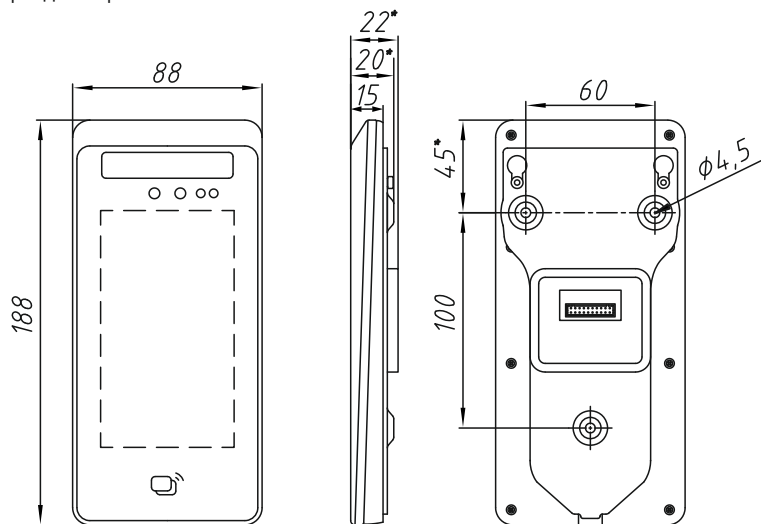
Рис. 1. Размеры и крепеж терминалов R20-Face (5W)
