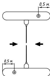
Рис. 6. Рекомендуемое размещение на турникете терминала R20-Face (8T) всех модификаций
